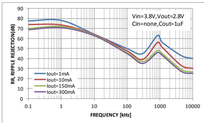
ME6211C28M5G
