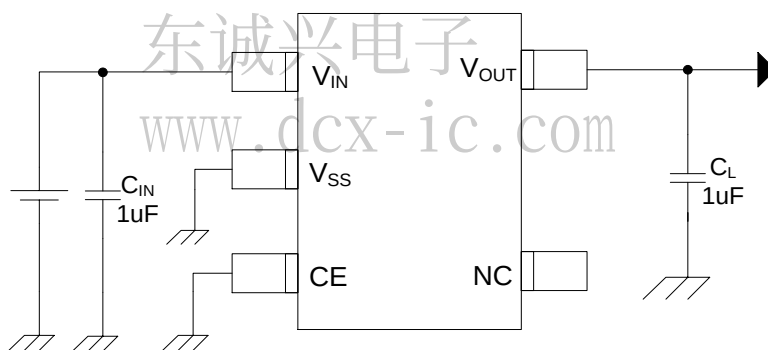
图 3. ME6211H 系列
