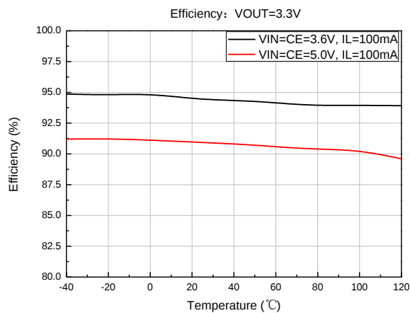
11、效率温度曲线
