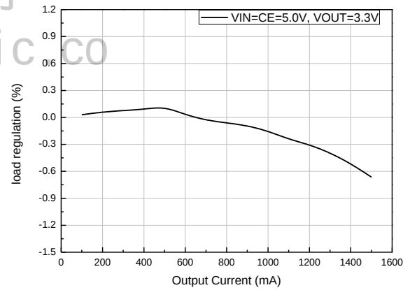
16、负载调整率 @ VOUT=3.3V
