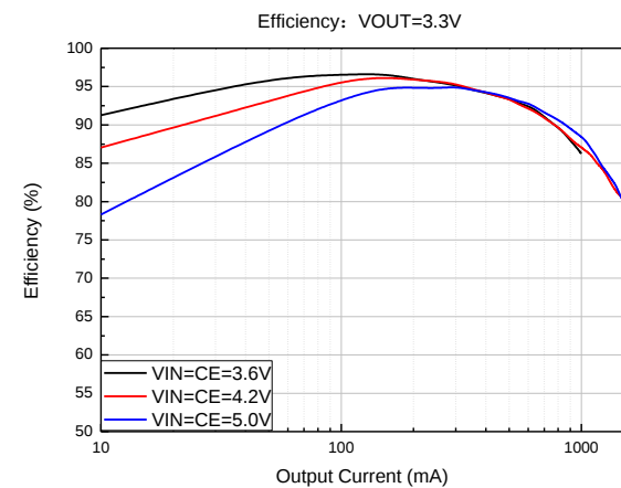
12、效率 @ VOUT=3.3V
