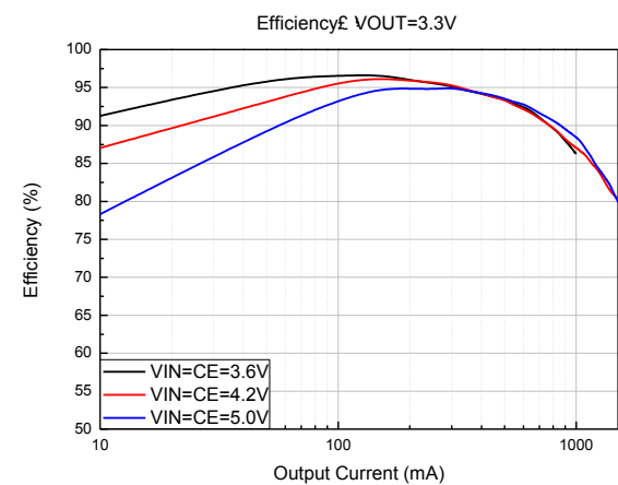
12、效率 @ VOUT=3.3V
